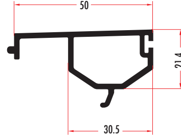
SIT7695 TEK RAYLI SÜRME KASA EŞİK KAPAMA PROFİLİ THRESHOLD PROFILE SIT7662 (RENKLİ/COLORED)
