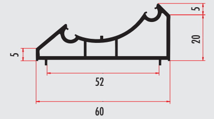
YARA601 60 MM KÖŞE DÖNÜŞ ADAPTÖRÜ CORNER ADAPTOR FOR 60 MM SERİE YARA602 (RENKLİ/COLORED)
