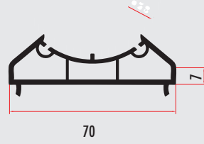
YARA701 70 MM KÖŞE DÖNÜŞ ADAPTÖRÜ CORNER ADAPTOR FOR 70 MM SERİE YARA702 (RENKLİ/COLORED)
